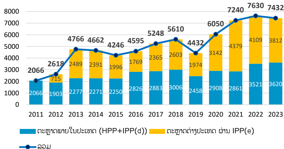
ການຜະລິດໄຟຟ້າຂອງ ຜ-ພຟລ ແຍກຕາມຕະຫຼາດ (GWh)
