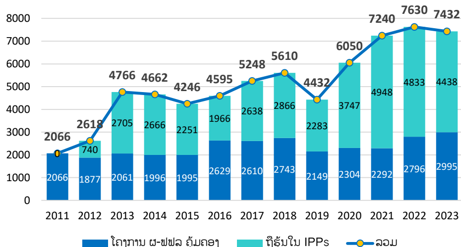
ການຜະລິດໄຟຟ້າຂອງ ຜ-ພຟລ ແຍກຕາມຕະຫຼາດ (GWh)
